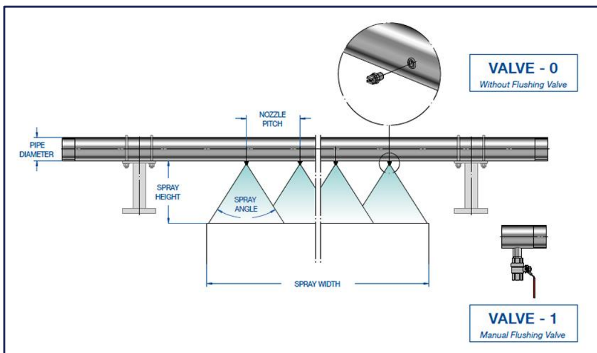
Rys.3. Natrysk niskociśnieniowy bez szczotki czyszczącej
