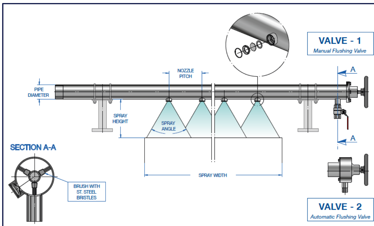
Rys.2. Natrysk niskociśnieniowy ze szczotką czyszczącą
