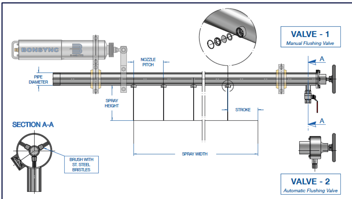
Rys 1. Natrysk wysokociśnieniowy ze szczotką czyszczącą
